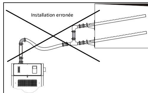
Illustration 13 - Tuyaux de distribution de vapeur : installation erronée
