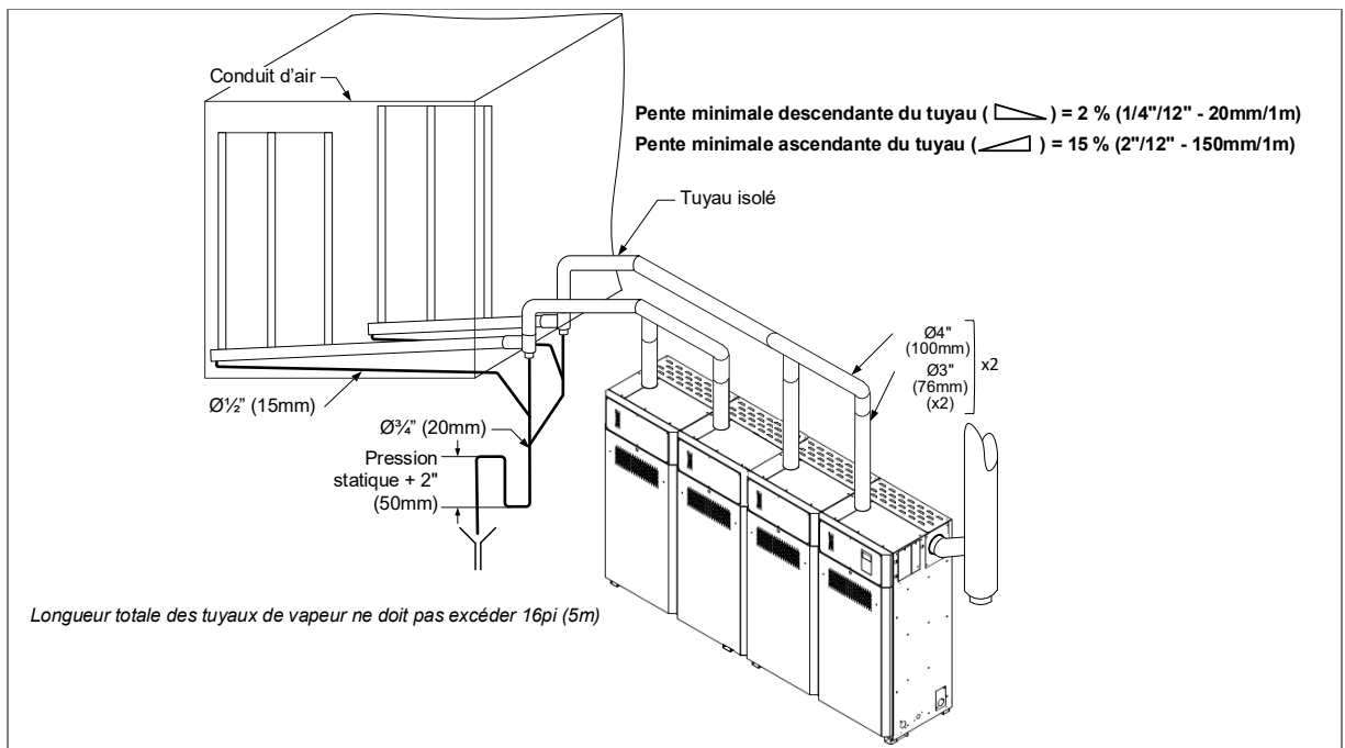
Illustration 26 - Tuyaux de vapeur Multi-Steam (SKG4-N7104 à 8104)
