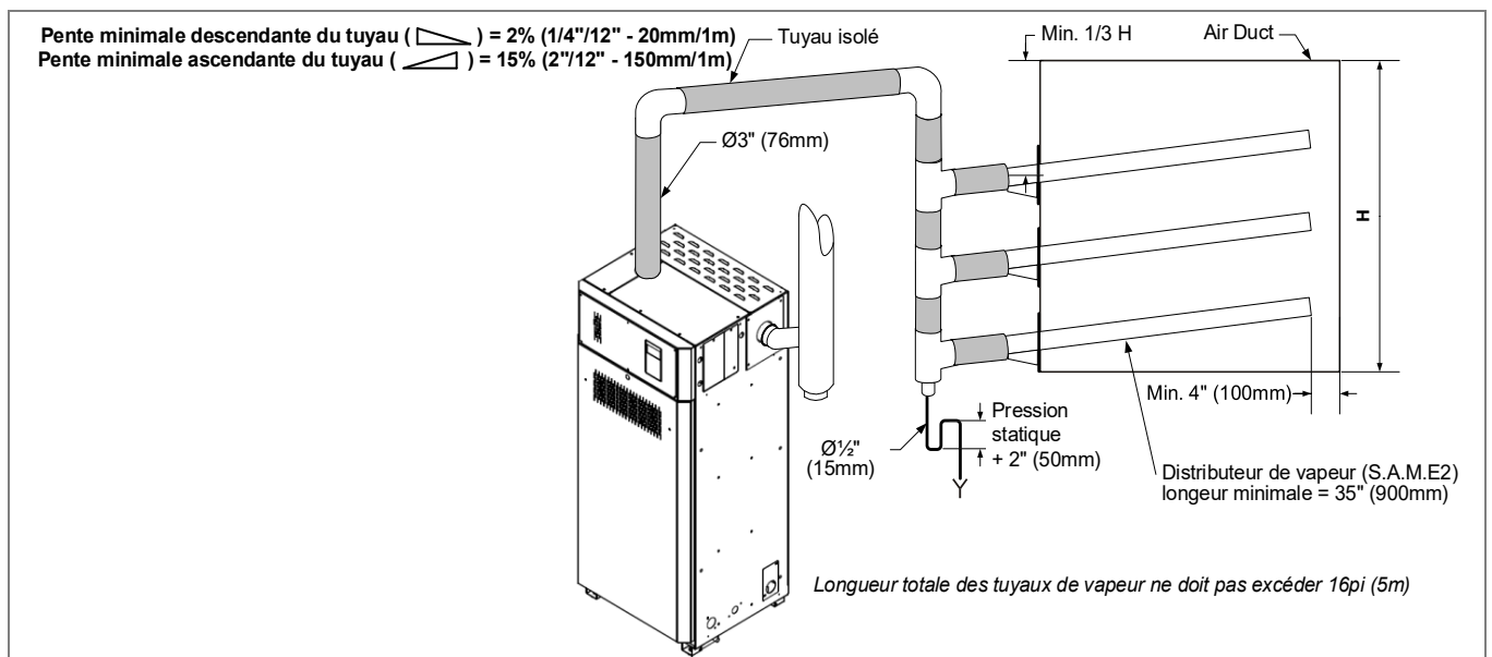
Illustration 20 - Tuyaux de vapeur S.A.M.E2 (SKG4-N1551 à 2101)
