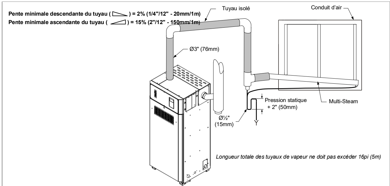
Illustration 23 - Tuyaux de vapeur Multi-Steam (SKG4-N1101 à 2651)
