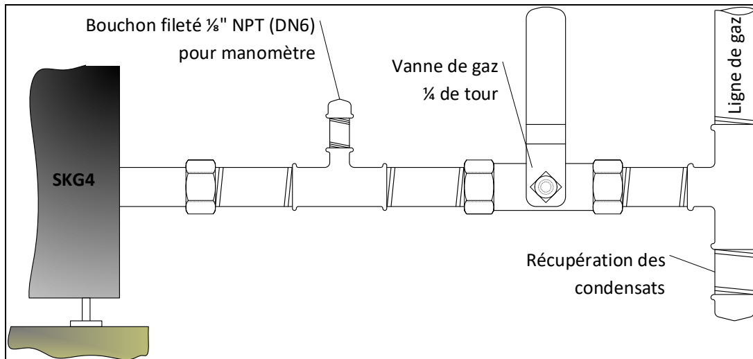
Illustration 27 - Alimentation en gaz
